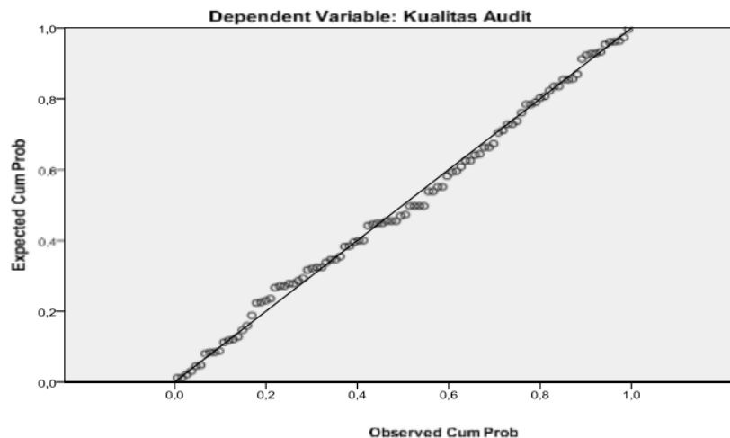
Gambar. 2 Uji Normalitas
