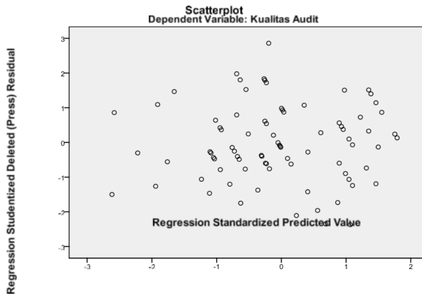
Gambar 3 Uji Heteroskedastisitas
