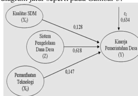
Gambar 3. Diagram Jalur Persamaan Substruktur 2
