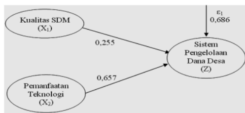
Gambar 2. Diagram Jalur Persamaan Substruktur 1
