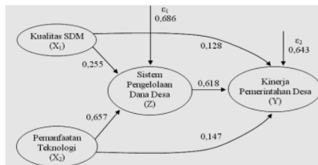
Gambar 4. Diagram Model Persamaan Dua Jalur
