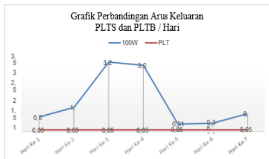
Gambar 7. Grafik perbandingan arus keluaran PLTS 100 WP dan PLTB/hari
