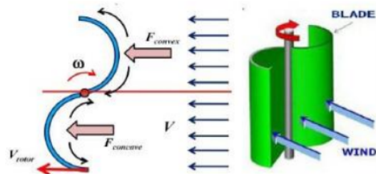
Gambar 1. Skematik turbin angin savonius dua sudut [6]
