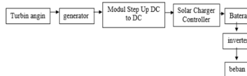
Gambar 4. Diagram Blok PLTB (Bayu/Angin)
