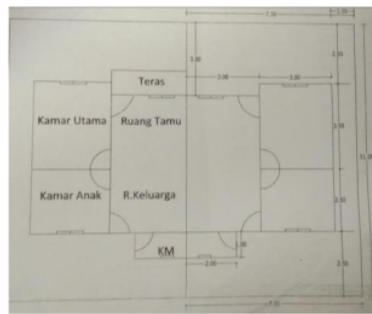
Gambar 1. Denah Rumah
