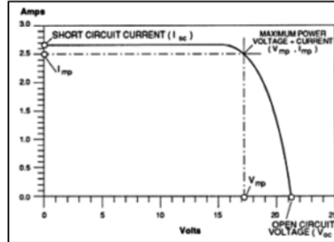
Gambar 4. Kurva Arus-Tegangan (I-V) Modul Surya
