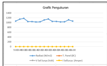
Gambar 7. Grafik Hasil Pengamatan Hari Kedua
