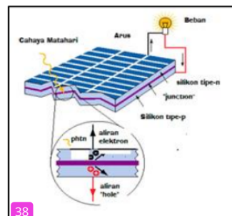
Gambar 2. Sel Surya Mengubah Energi Matahari Menjadi Listrik
