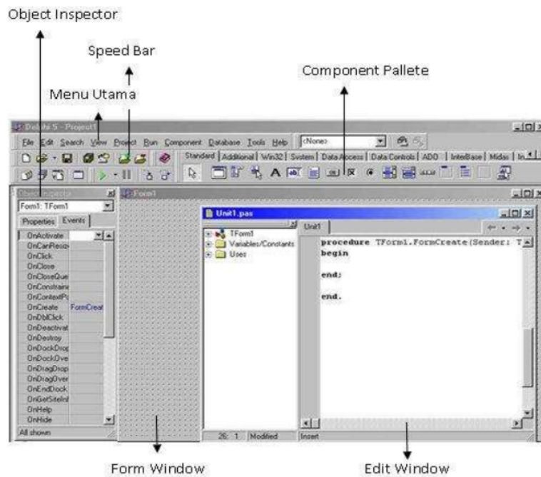
Gambar 1. Tampilan IDE Borland Delphi 5.0
