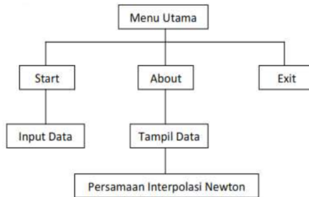
Gambar 2. Struktur Program
