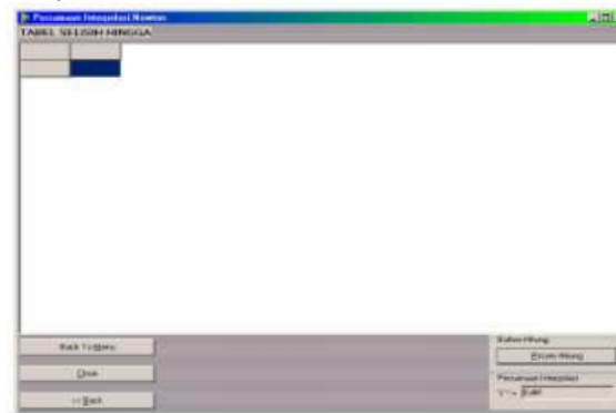
Gambar 12. Form persamaan interpolasi newton
