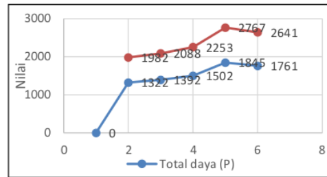
Gambar 4. Grafik Hasil Perhitungan Daya, Energi Listrik pada Motor Induksi Hubungan Delta tanpa Beban
