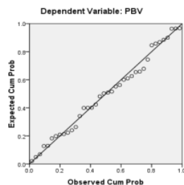
Gambar 1. Pengujian Normalitas
