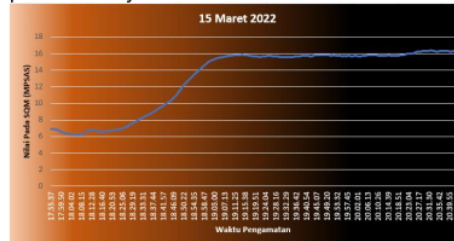
Gambar 1. Grafik SQM tanggal 15 Maret 2022 dari jam 17.55 – 20.40 WIB
