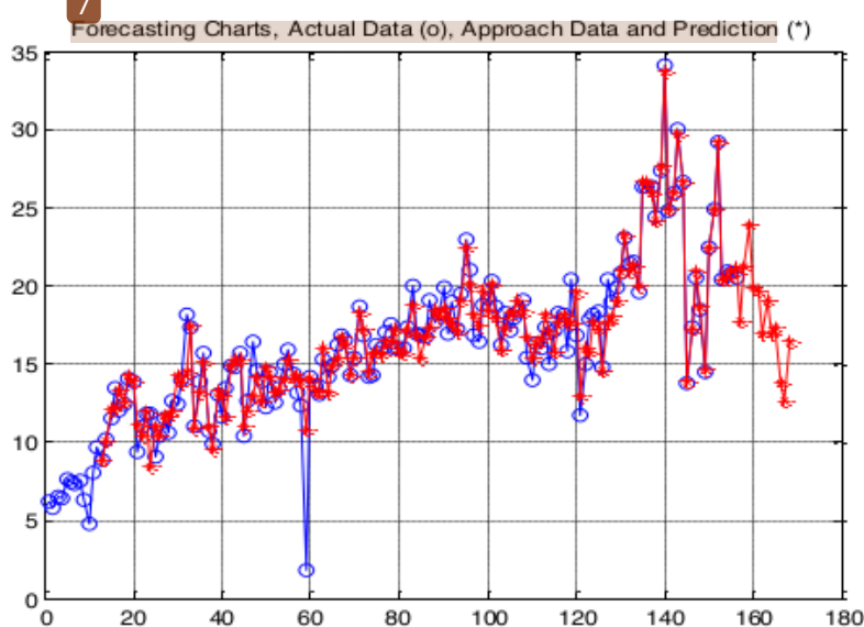
Gambar 2. Pendekatan data forecasting dan data actual
