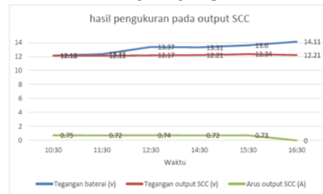
Gambar 3. Grafik Hasil Pengukuran Output SCC
