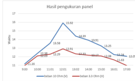
Gambar 2. Grafik Hasil Pengukuran Panel Surya
