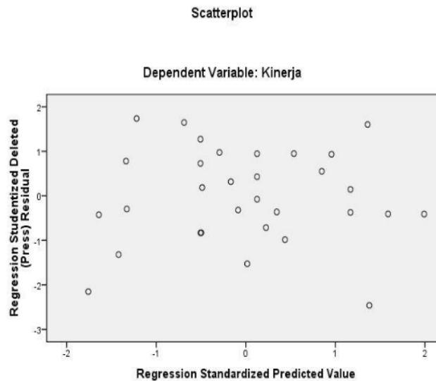
Gambar 4.4. heterokedastisitas
