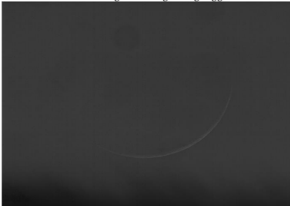
Gambar 12 Hilal setelah Matahari terbenam
