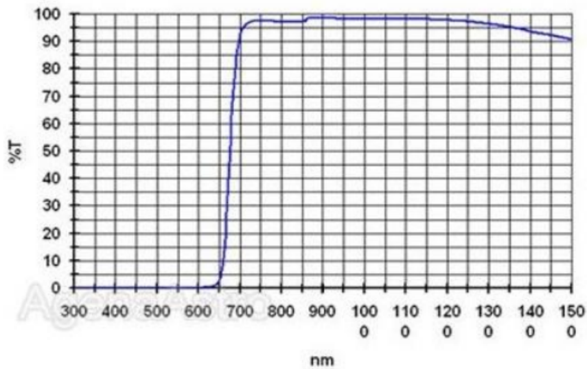
Gambar 5 Sensitivitas spektrum filter Baader IR
